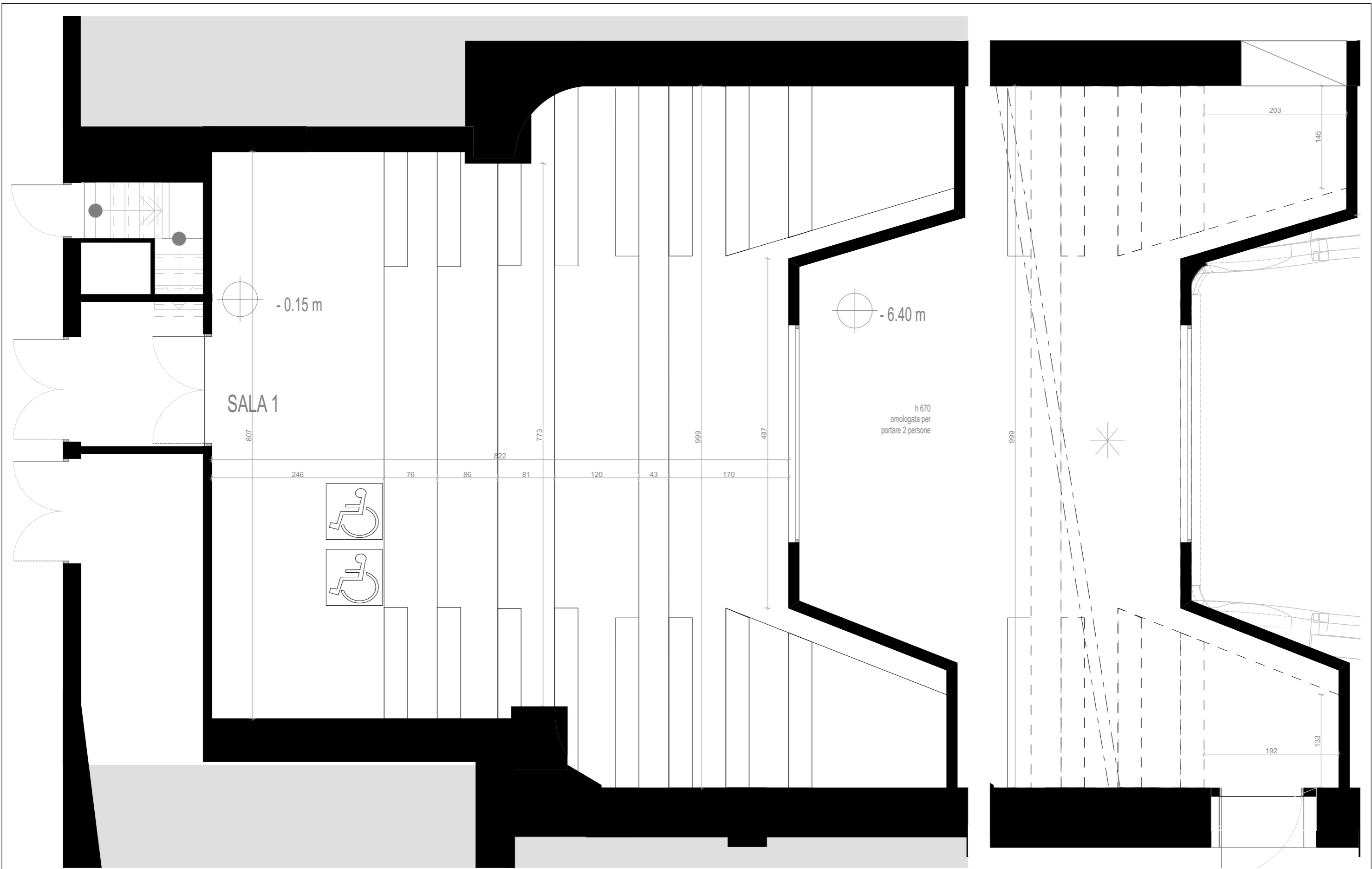
Pianta galleria - piano terra
